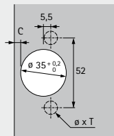
Πλήρες πάτημα (Βάση B 11.5 mm)
